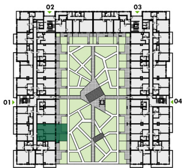
PŮDORYS PODLAŽÍ
